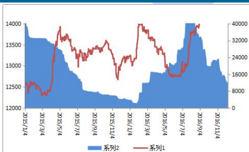
现货铅于 SHFE 铅库存走势图
