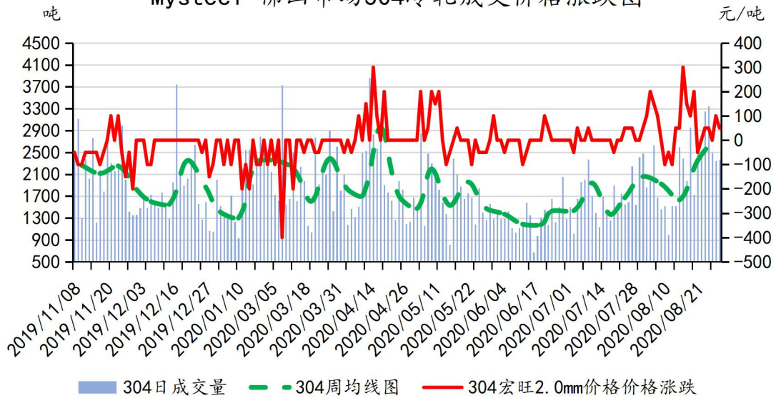
Mysteel-佛山市场304冷轧成交价格涨跌图
