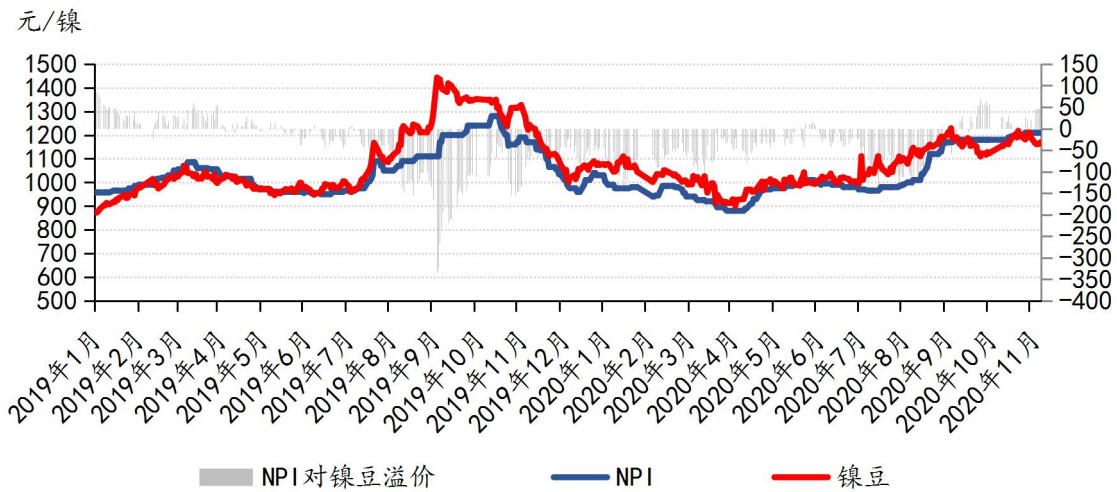
Mysteel-NPI与镍豆经济性对比
