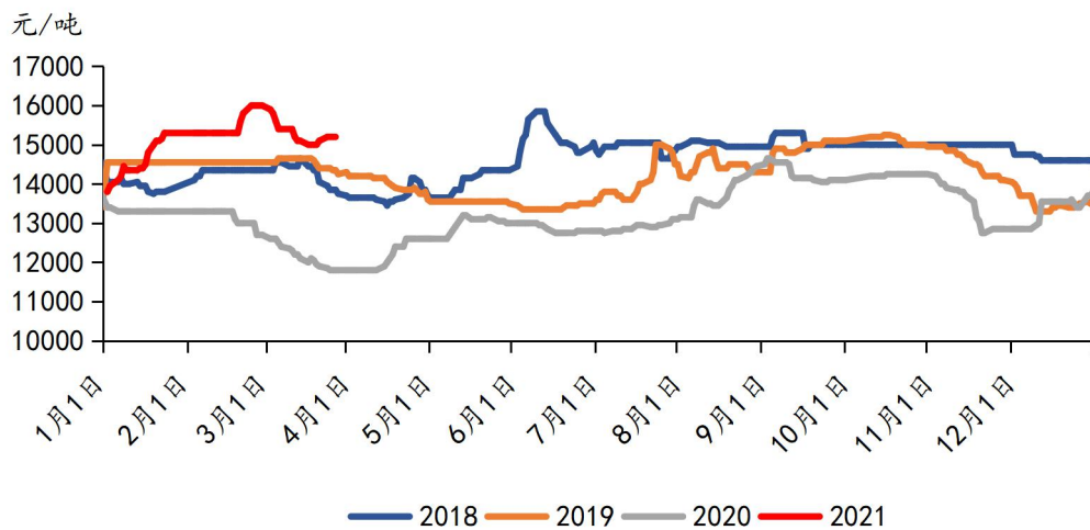
Mysteel-北部湾新材: 佛山市场价格: 304/NO.1
