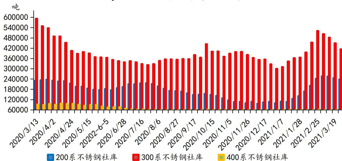
Mysteel-不锈钢分系别社库
