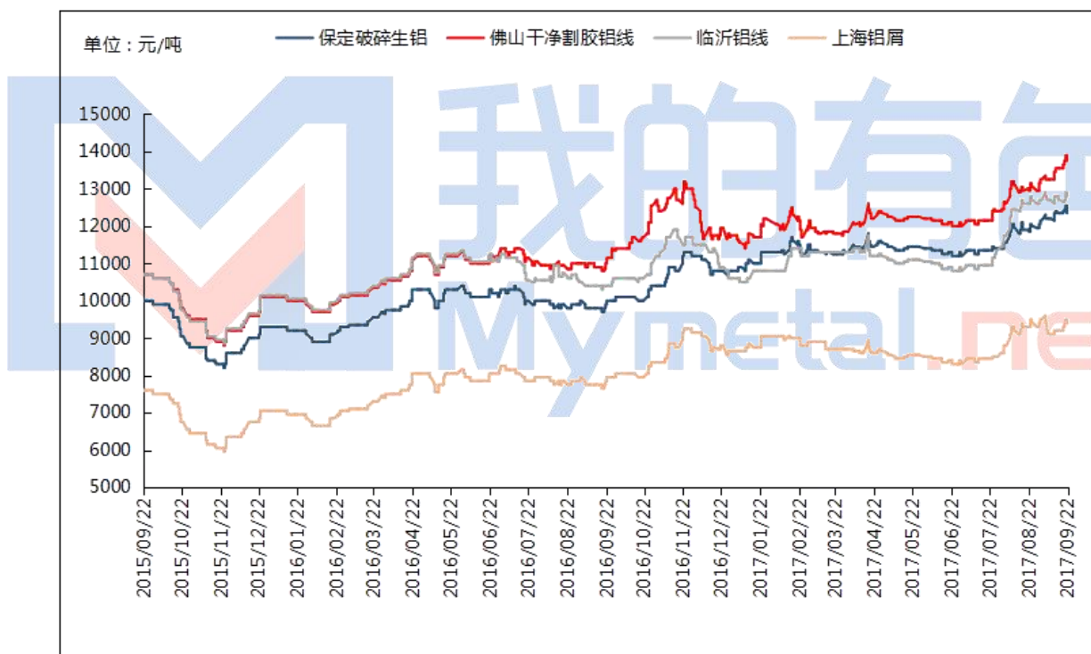
图2 国内废铝价格走势
