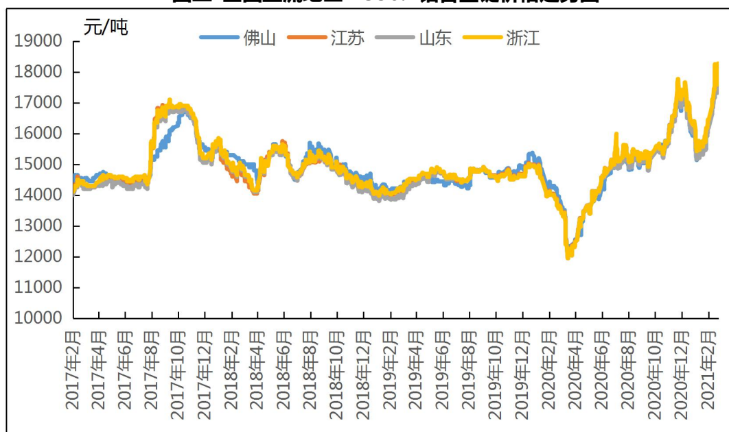
图三 全国主流地区 A356.2铝合金锭价格走势
